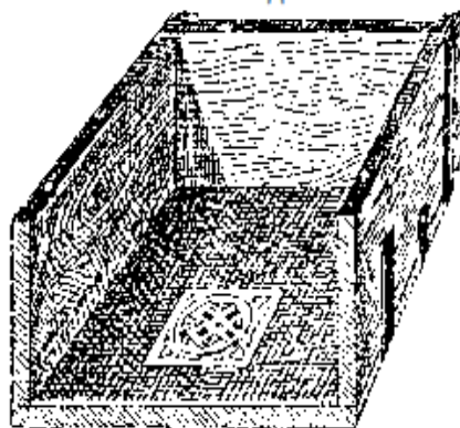
Рис. 4. Разъемная форма для сырца
